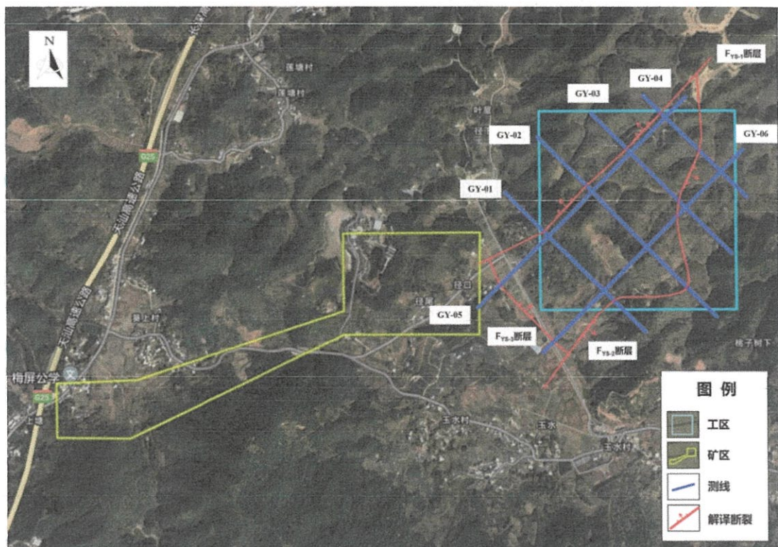
图 3-1 工区断层解译平面图
