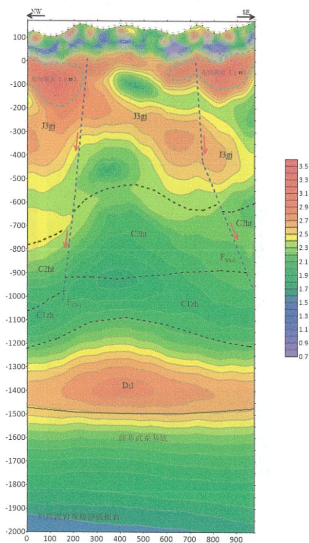
图 3-4 断层要素
